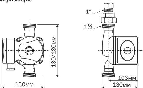
Габаритные размеры
